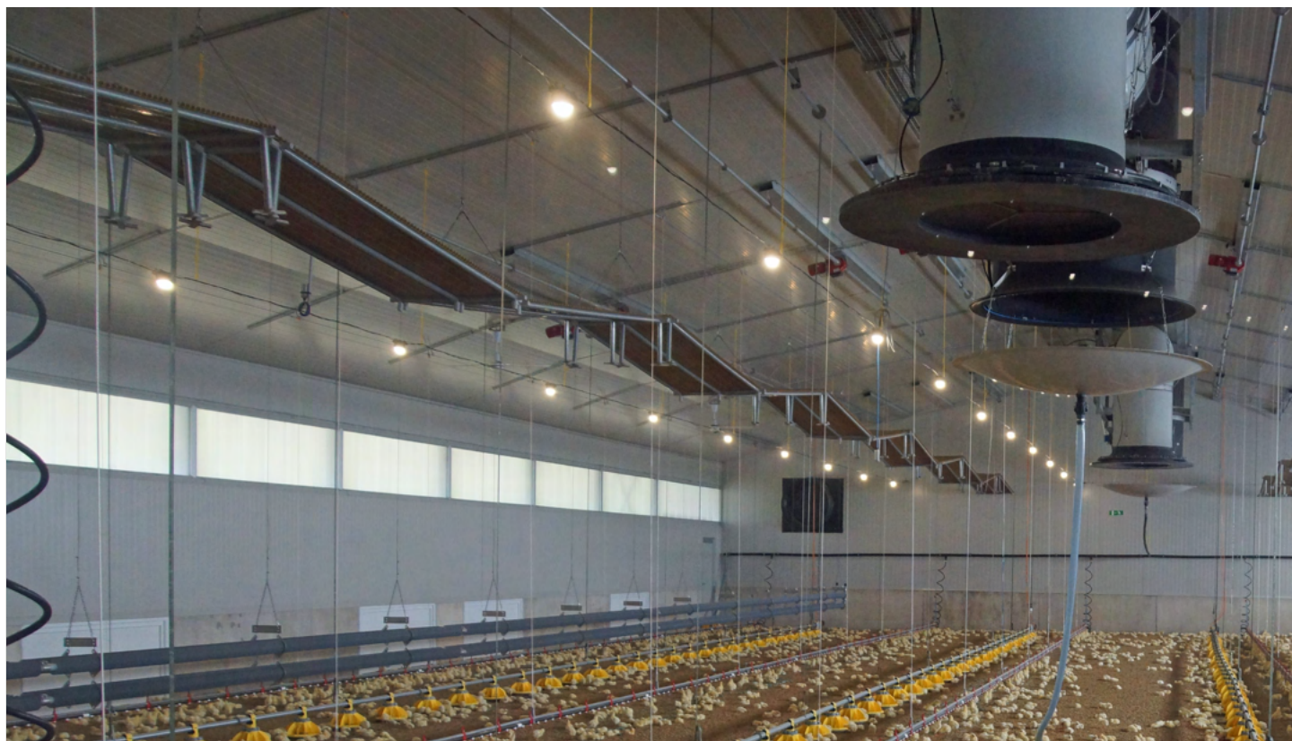
Die Wärmeverteilung erfolgt in Hellsau über frei hängende Rippenrohre (2 Bahnen à je 4 Rohre links und rechts im Stall). Im Vordergrund ersichtlich ist ein Zuluftverteiler, welcher sicherstellt, dass die vorgewärmte Luft auch in die hinterste Stallecke gleichmässig verteilt wird; die Abluft entweicht über die zwei Rohre in der Mitte des Daches. Foto: Marianne Etter
